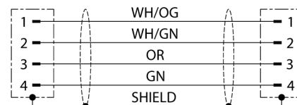
Schéma zapojení
